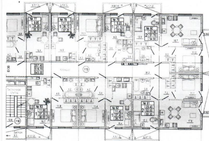
Литер - 2, БС - 1, 7 этаж, кв. 80
