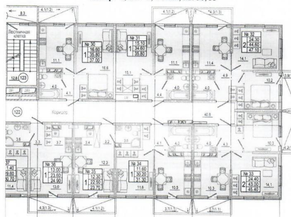
Литер - 1, БС - 1, 4 этаж, кв. 30, 33
