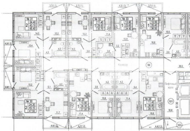
Литер - 2, БС - 1, 4 этаж, кв. 30
