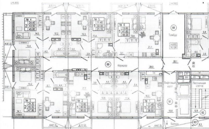
План Литер - 2, БС - 1, 2 этаж, кв. 4
