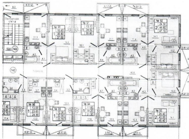
Литер - 1, БС - 1, 8 этаж, кв. 92
