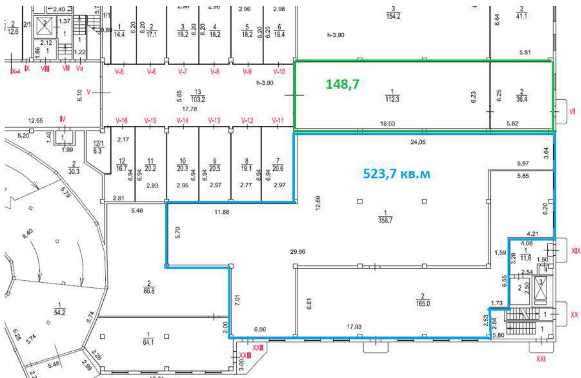
Рис. 4. Схема оцениваемых помещений на плане этажа №1
